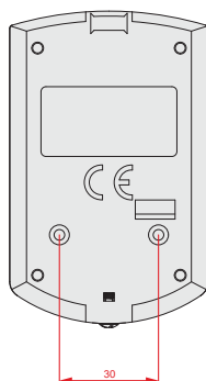
XIRP100H - back
